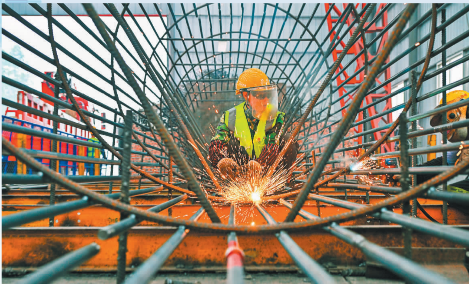
▶6月1日,四川省眉山市仁寿县禄加镇的资乐高速公路2号预制梁场,施工人员进行焊接。潘帅摄(中经视觉)
