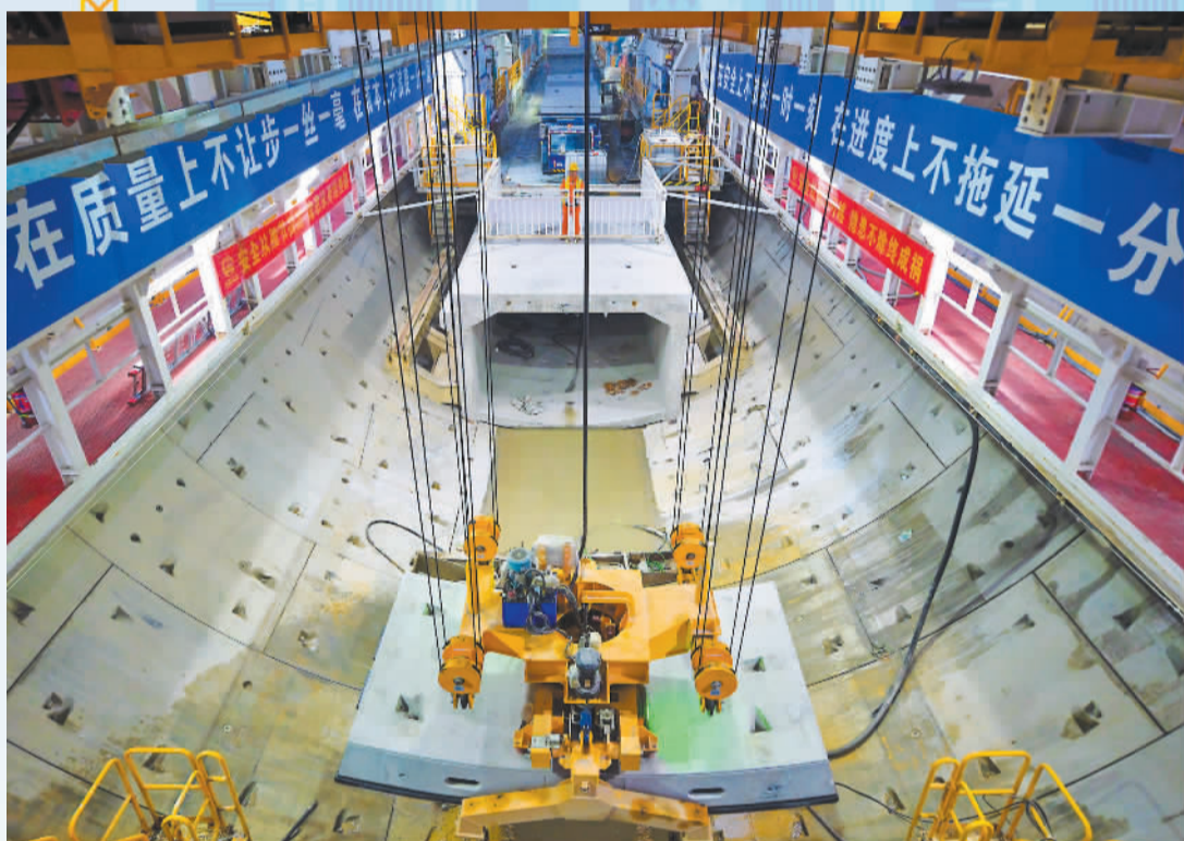
▲5月21日,在浙江省杭州市萧山机场西隧道盾构区间,技术人员正在进行吊装管片作业。刘玉才摄(中经视觉)
