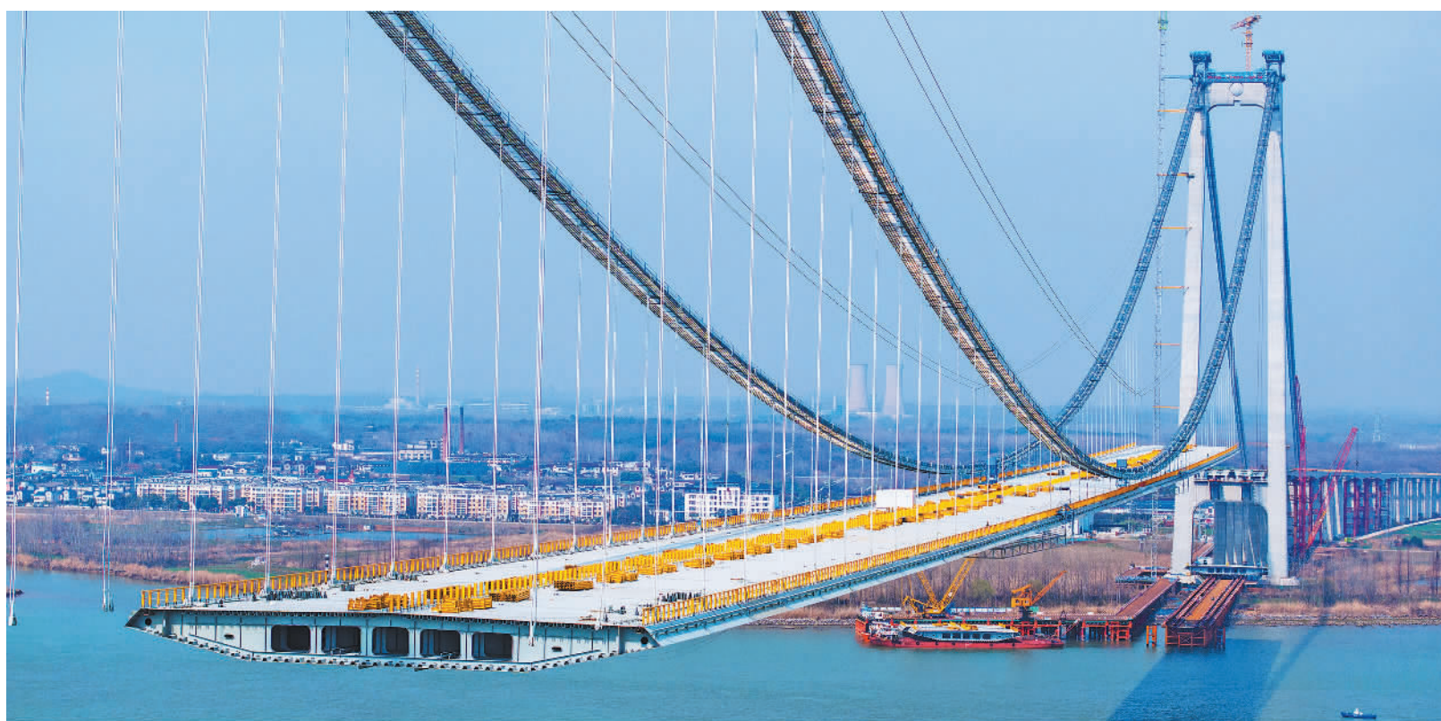
2月26日,建设中的龙潭长江大桥。该桥北接江苏扬州仪征市,南接南京市、镇江句容市,目前已进入钢箱梁吊装施工阶段,预计今年3月底吊装完成。大桥建成后,将对当地加快构建区域综合立体交通走廊、优化过江通道布局、完善高速公路网络等发挥积极作用。方东旭摄(中经视觉)
