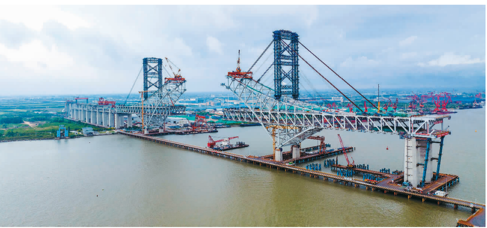
6月24日，中交二航局建设者在常泰长江大桥5号索塔上作业。为应对高温天气，工地调整作息时间，避开高温错峰作业，确保作业人员安全。常泰长江大桥连接江苏常州和泰州两市，全长10.03公里，是一座集高速公路、城际铁路和普通公路为一体的过江通道。汤德宏摄(中经视觉)
