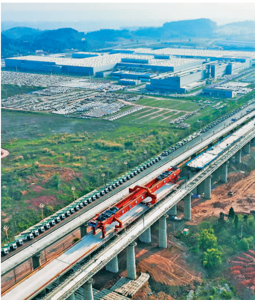
图为1月28日，在四川宜宾三江新区建设中的渝昆高铁、成自宜高铁宜宾段沙坪坝多线特大桥。这是渝昆高铁与成自宜高铁四线并行的特大桥，也是两条高铁宜宾段全线的控制性工程。渝昆高铁建成后将成为西南地区对外开放大通道。成自宜高铁建
