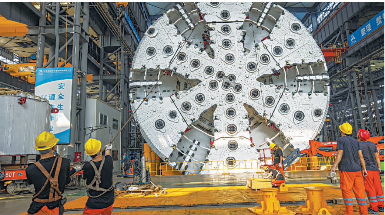
8月24日,广东省佛山市顺德区的中铁华隧联合重型装备公司盾构机生产车间内,工人们正在吊装大型盾构机刀盘。该盾构机直径为15.56米,总重4300吨,计划8月底下线交付客户,将应用于佛山季华路西延线工程建设。付海燕摄(中经视觉)
