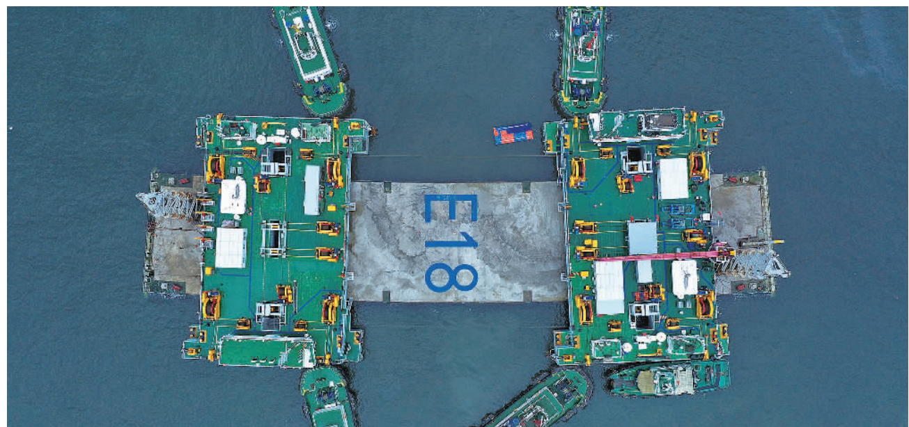
近日,我国北方首条大型跨海沉管隧道——大连湾海底隧道最后一节沉管顺利完成安装。至此,大连湾海底隧道沉管安装任务全部完成。隧道建成后将成为纵贯南北的快速通道,推动大连湾一体化建设。田晋江摄(中经视觉)
