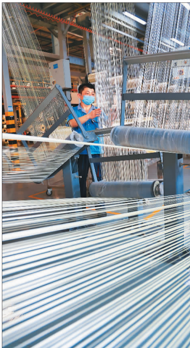
▼江苏省连云港经济技术开发区中复神鹰碳纤维股份有限公司,工人在碳纤维生产线上忙生产。 耿玉和摄(中经视觉)
