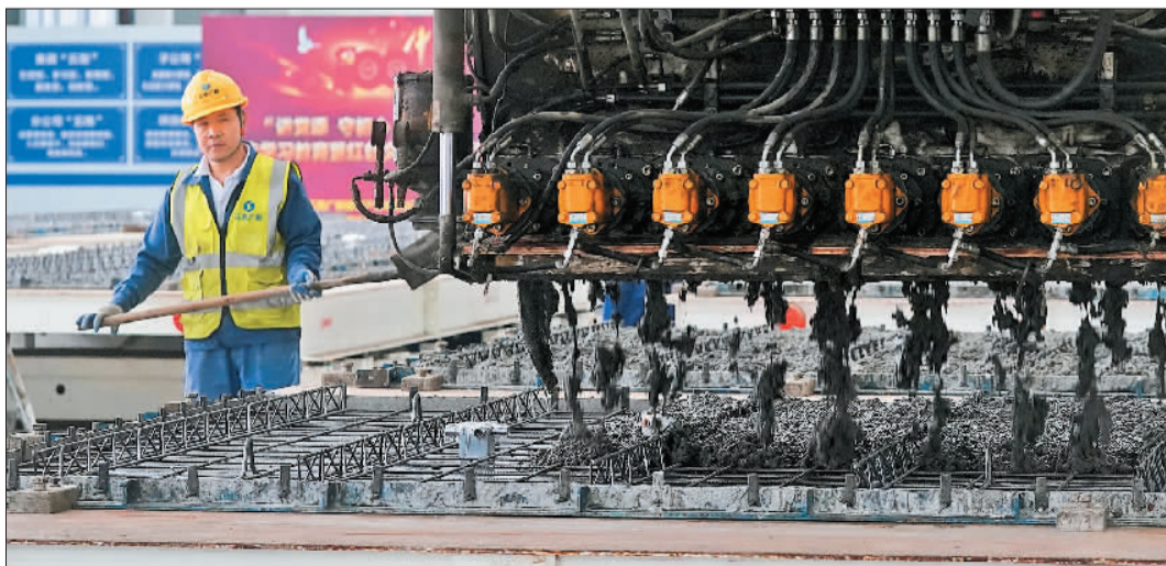
▼江西广新建筑产业有限公司PC构件生产车间,工人在赶制装配式建筑材料。江西省大力发展装配式建筑,2022年全省装配式建筑目标新开工面积达到总建筑面积的30%。 徐云摄(中经视觉)
