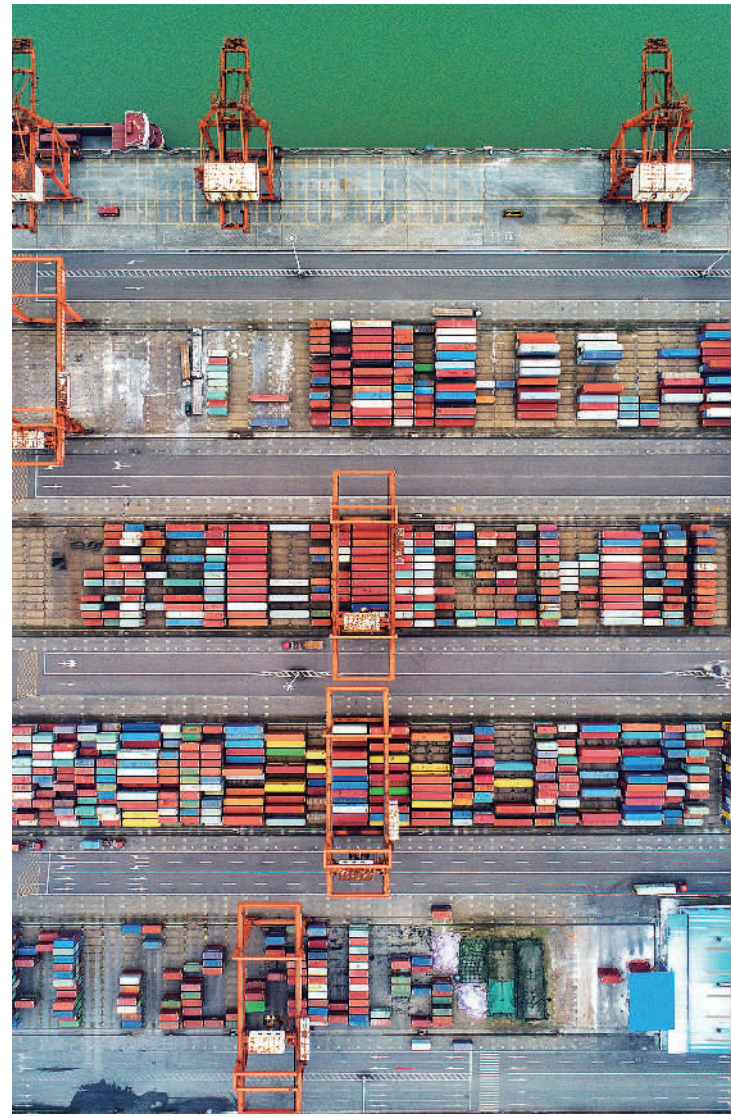
11月15日，位于四川省宜宾市三江新区的宜宾港集装箱码头，船舶、集装箱卡车正有序作业。日前，川南港务公司宜宾港5G智慧港口一期项目完成初步验收，并上线试运行。宜宾港通过港口集装箱作业管理、集装箱智能闸口以及港口业务大数据可视化三套智能系统，由传统码头改造升级为智慧码头。 庄歌尔摄(中经视觉)
