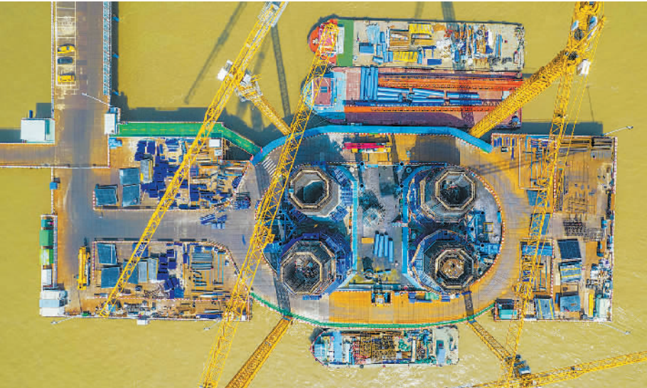
10月1日，在江苏泰州常泰长江大桥建设工地，工人正对5号墩主塔下塔柱进行钢筋绑扎施工。 汤德宏摄(中经视觉)
