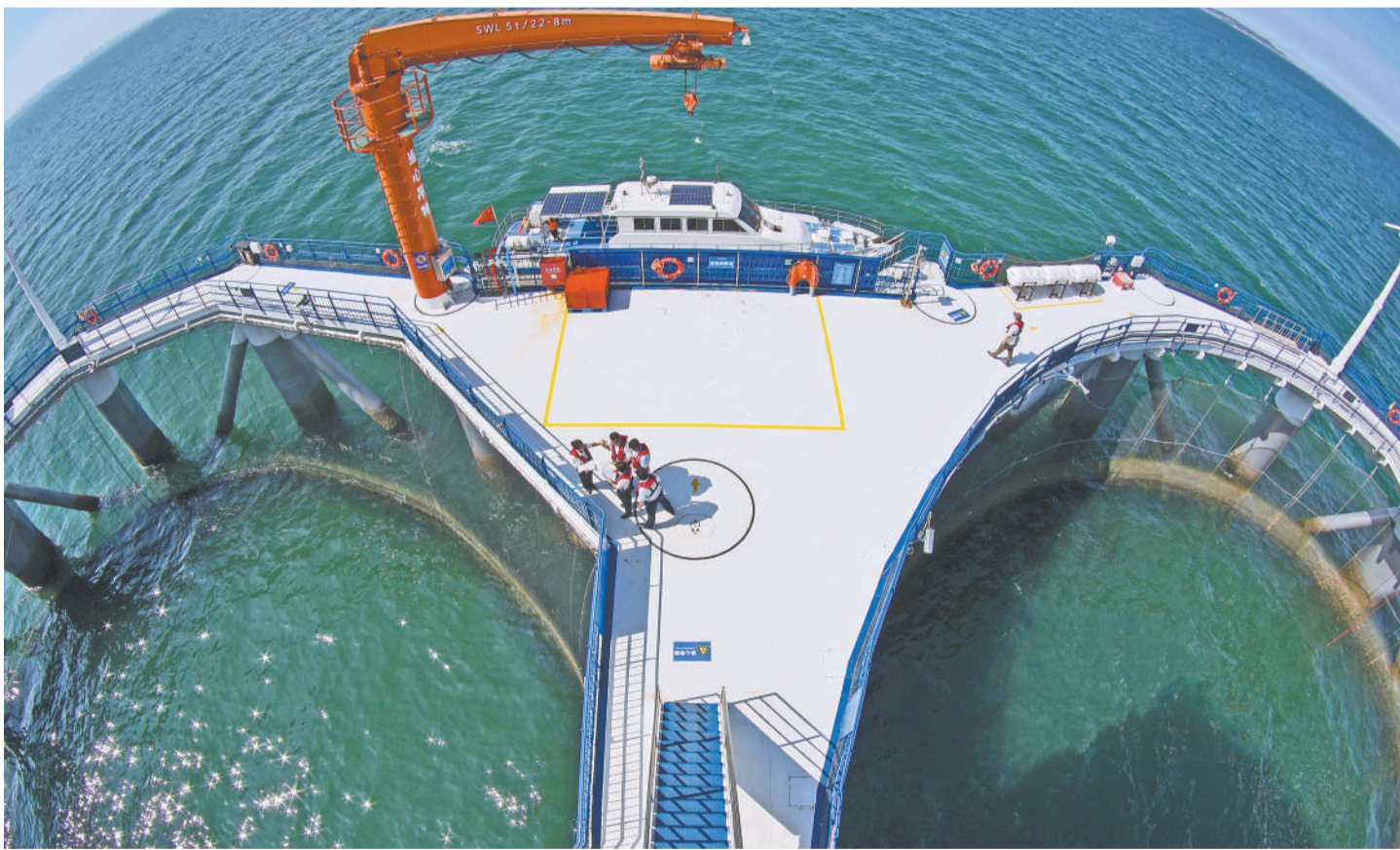
7月27日,山东烟台四十里湾海域的“耕海1号”海洋牧场综合体平台顺利通过海关注册登记评审,成为全国首家注册出境水生动物养殖场成功的装备型海洋牧场。该平台配备了自动投饵、环境监测、大数据分析、5G通信、安全管理等系统,通过科技创新提升海洋渔业精细化管理水平。唐克摄(中经视觉)
