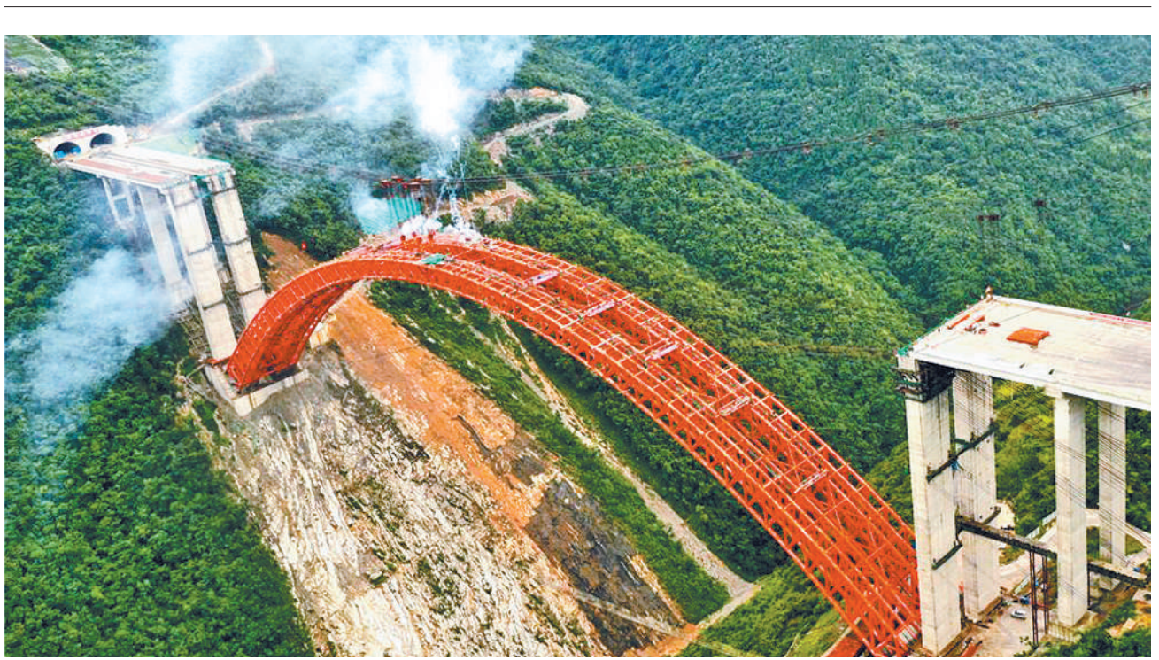
7月27日,由贵州桥梁集团承建的仁(怀)遵(义)高速公路主要控制性工程——大发渠特大桥主拱顺利合龙。大发渠特大桥位于贵州省遵义市播州区和汇川区境内,全长1427米、主跨410米、桥宽33米。 本报记者 吴秉泽摄
