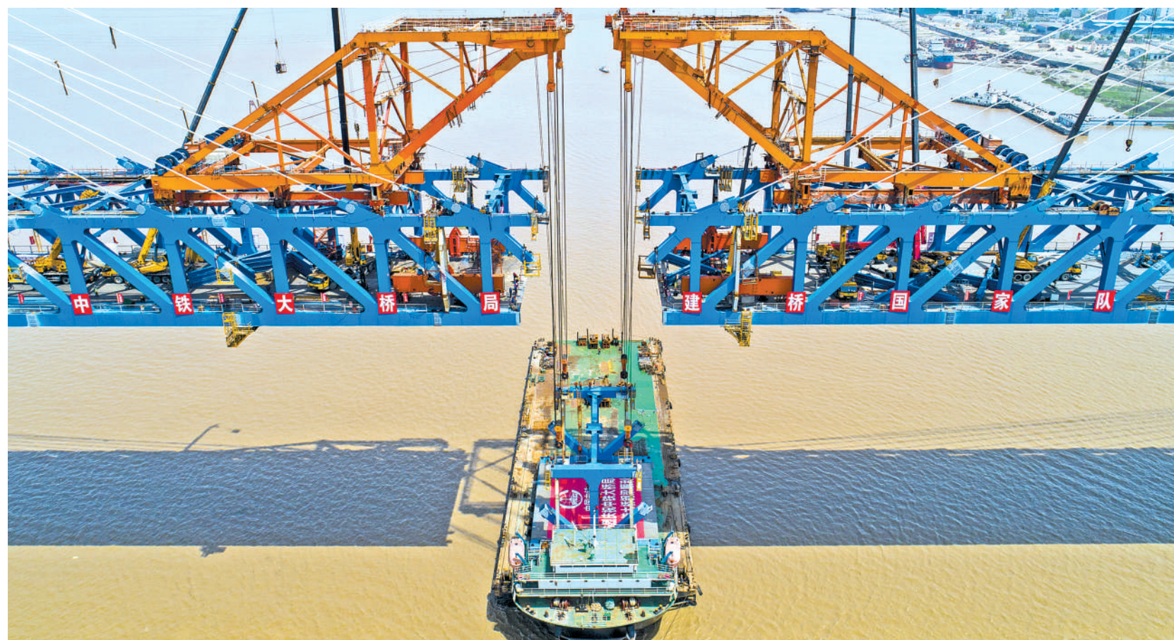
四月十七日,杭绍台铁路椒江特大桥合龙现场(无人机照片)。当日,在浙江台州,杭绍台铁路是我国首条民营资本控股的高速铁路项目,该线路连接浙江杭州、绍兴和台州三地,线路设计时速三百五十公里。孙金标摄(新华社发)
