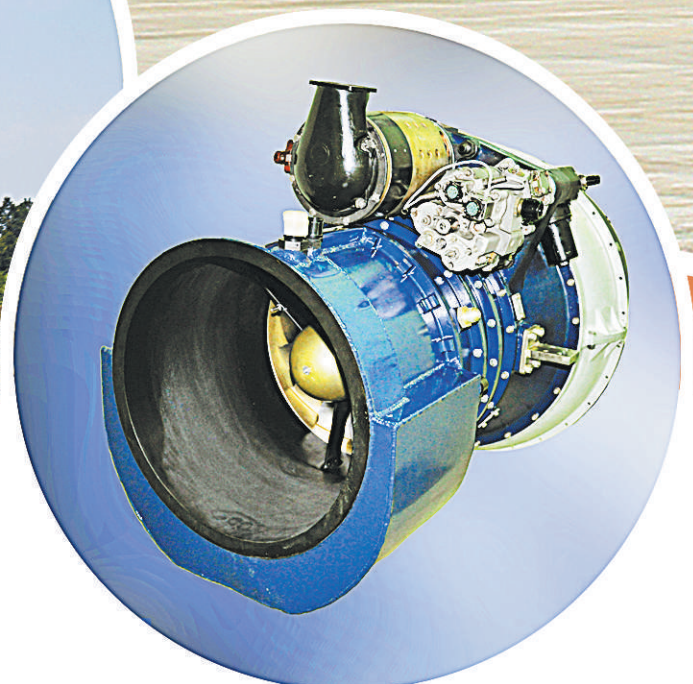
中发天信研发的小型航空发动机
