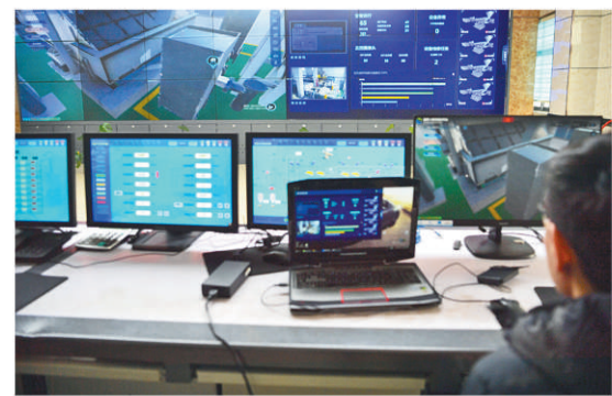
鲁西煤矿智能化洗煤厂集控中心。
