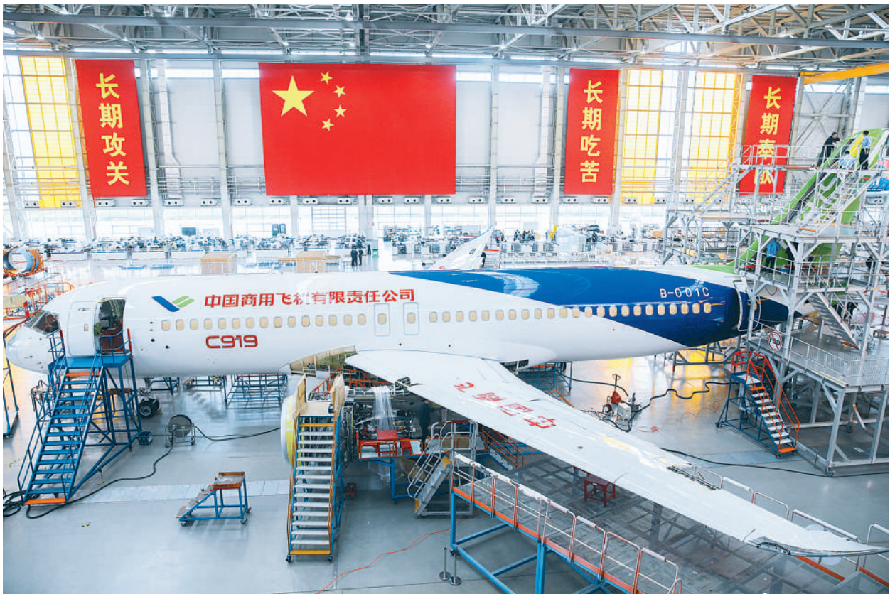
C919大型客机102架机停放在中国商飞公司上海飞机制造有限公司总装车间内(10月18日摄)。 10月18日,记者来到中国商飞公司上海飞机制造有限公司总装车间,探秘C919大型客机102架机。据悉,C919大型客机102架机已于10月11日完成整机喷漆工作,目前正在进行发动机安装调试、试飞测试系统改装和开车前的地面功能检查试验等工作,计划近期推出总装厂房,开展外场功能试验。 新华社记者 丁 汀摄
