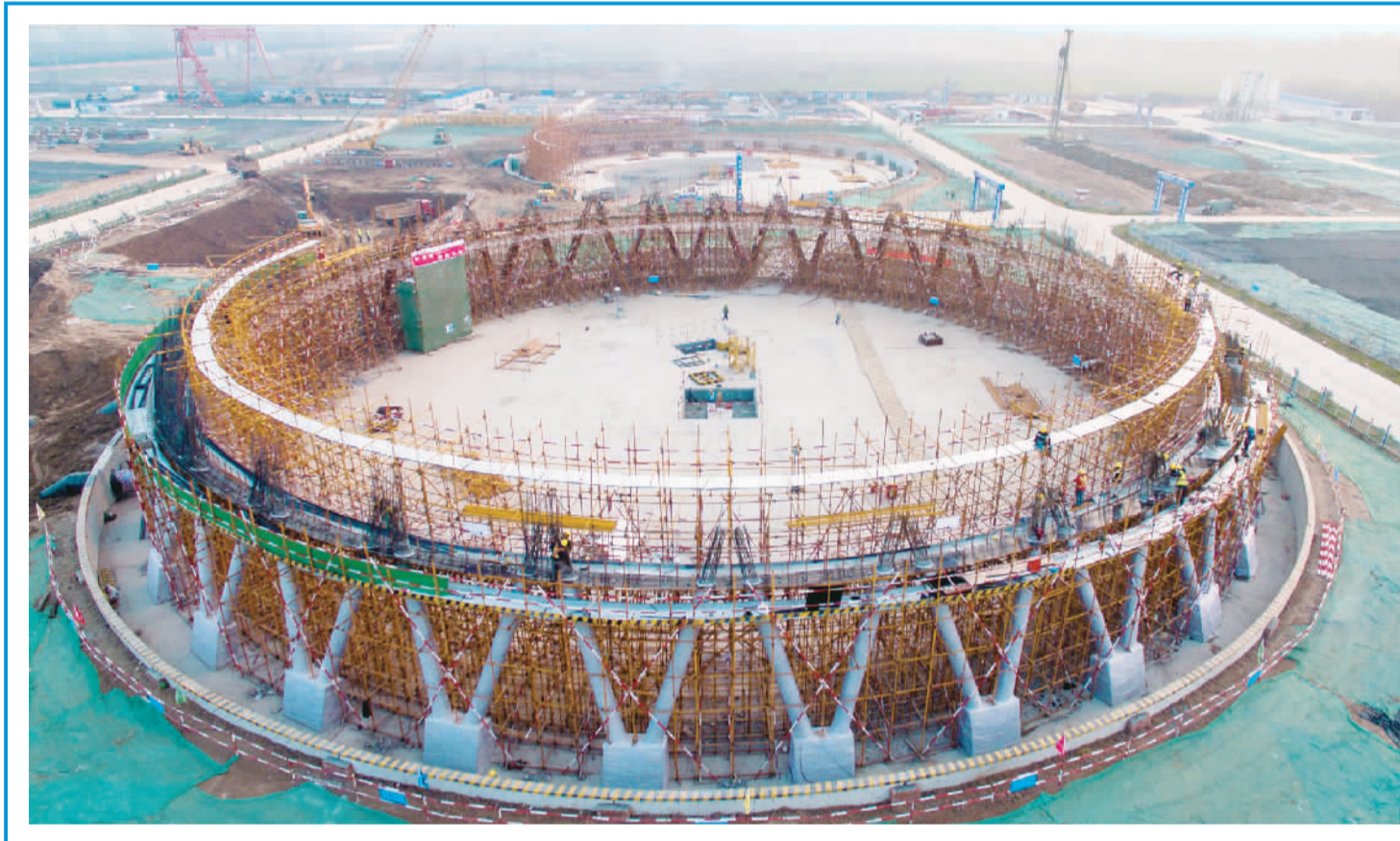
这是12月18日拍摄的河南项城2×300MW等级燃气—蒸汽循环发电项目工地。该项目总投资28.8亿元,近日正式开工,是国家“西气东输一线”总体规划中的重要燃气发电工程,也是河南省“十三五”重点建设工程。据悉,该项目利用天然气清洁能源实行热电联产,兼顾电网调峰和管道调峰,项目建成后年发电量36亿千瓦时,年供热量640万吉焦。 时初鹏摄
