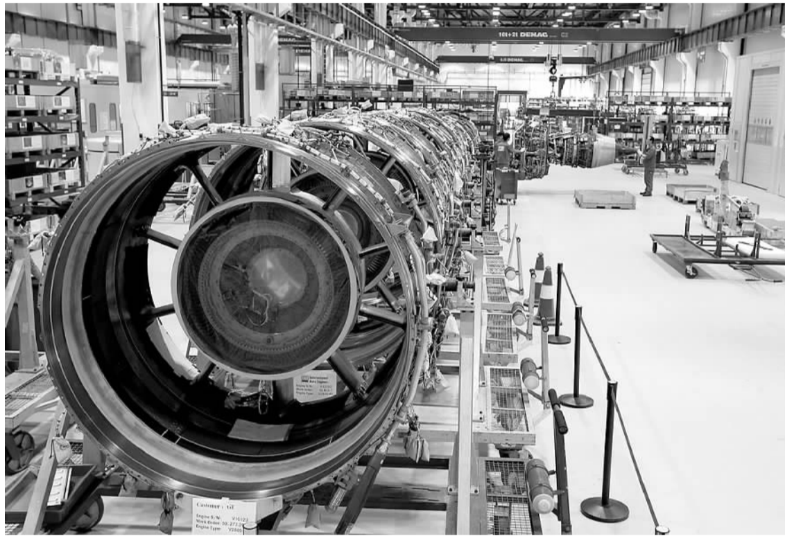
图为位于珠海保税区的摩天宇航空发动机维修有限公司车间。摩天宇、翔翼等一批企业为珠海航空类企业增强发展全面性、协调性和可持续性提供了重要的配套支撑。(资料图片)
