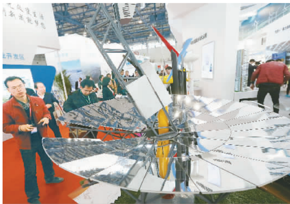
3月29日,在一个绿色能源展台,参观者在观看蝶式斯特林光热发电模型。当日,为期3天的第八届中国国际清洁能源博览会在中国国际展览中心开幕。本届博览会以“中国清洁能源‘十二五’总结与‘十三五’展望”为主题,聚焦各类清洁能源产品及相关技术。
