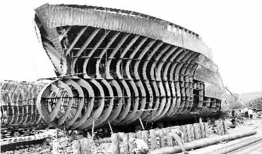
因为重庆云阳县河牛航运公司的造船码头,工人们正在忙着建造数重量7600吨的滚装船。
