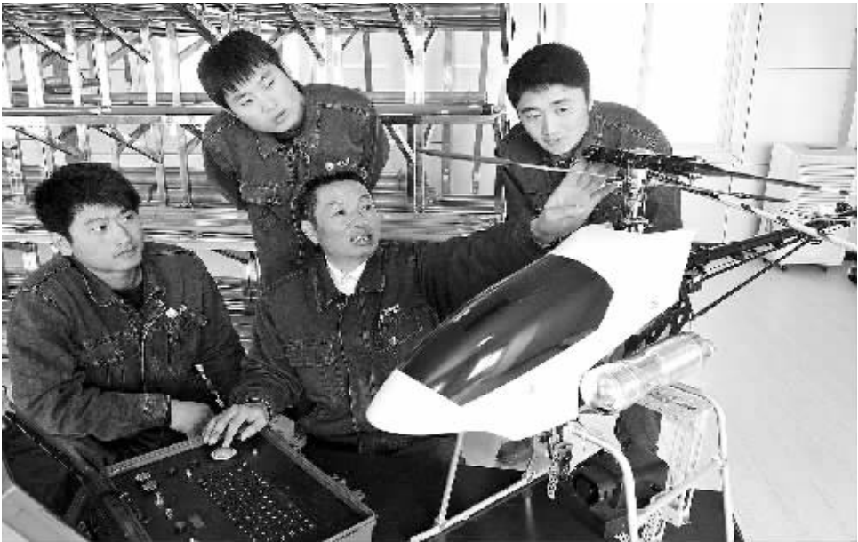
许启金(右二)向徒弟们讲解无人机巡线技术。
