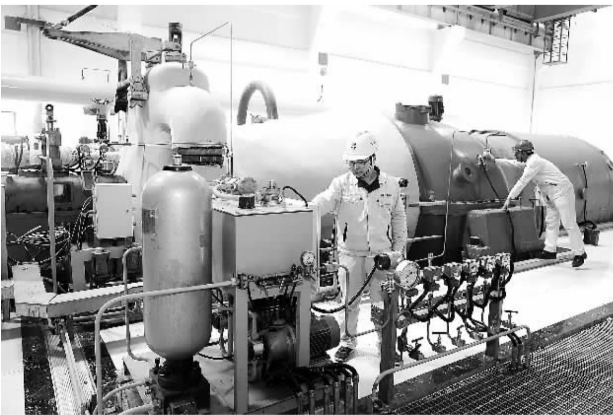
工作人员对华电九江分布式能源站汽轮机发电设备进行试运行前检查。3月17日，江西第一个工业园分布式能源示范项目——华电九江分布式能源站在江西九江市城东港区试运营。该能源站的投入运行，预计每年可减排二氧化碳7411万吨、氮氧化物5682吨和烟尘9200吨。
