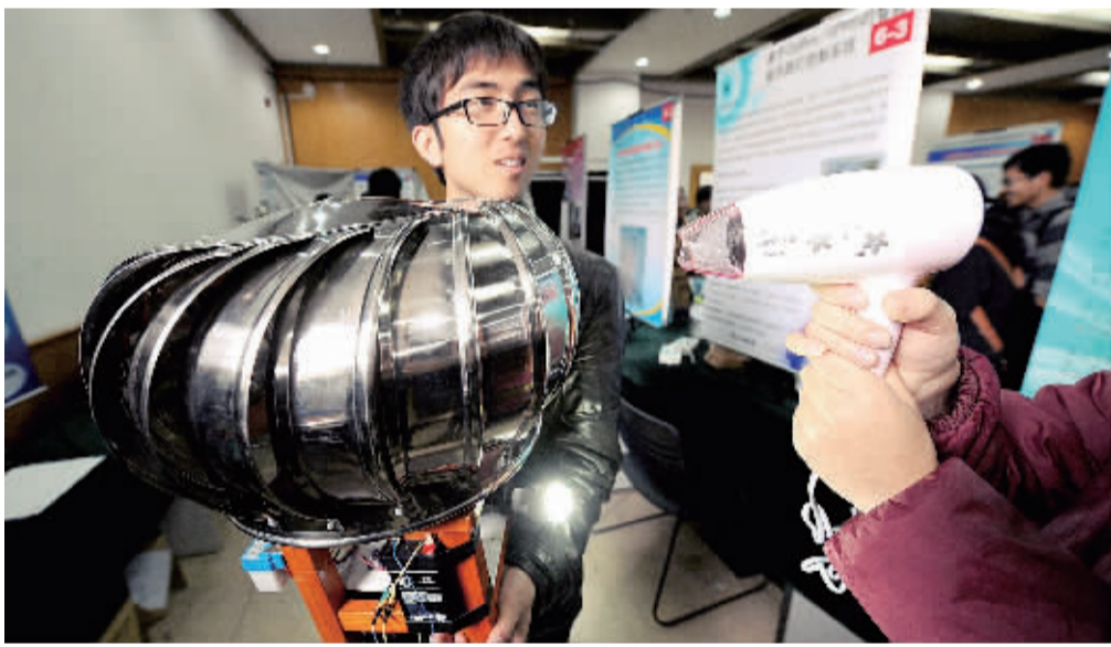
11月23日,来自东南大学吴健雄学院的参赛学生在演示其研制的“垂直轴风力发电、储能与照明装置”。当日,江苏省大学生物理及实验科技作品创新竞赛在南京东南大学举行,省内42所高校的学生选手携234项作品参加决赛并进行展示。新华社记者 孙 参摄
