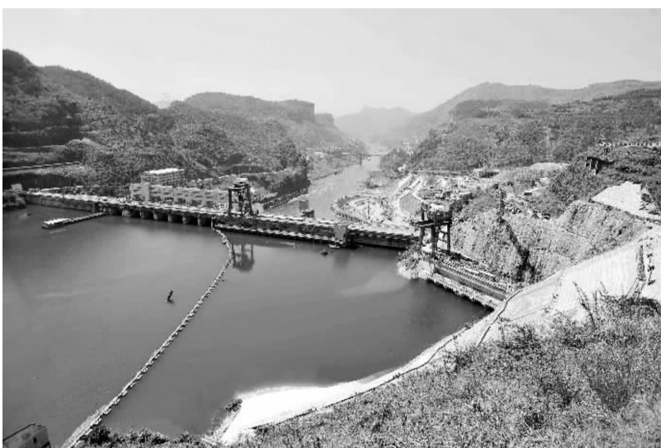
这是正在加建二期工程的岩滩水电站,右岸是建设中的二期工程入水口(6月14日摄)。目前,工程人员正在紧张修建位于广西壮族大化县境内的岩滩水电站引水发电系统工程。岩滩水电站是红水河梯级开发方案的第五级水电站,其二期工程于2010年10月正式开工,增建两台300兆瓦混流式水轮发电机组。按原定计划2014年6月工程竣工后,岩滩水电站装机容量将增至1810兆瓦。新华社记者 张爱林摄
