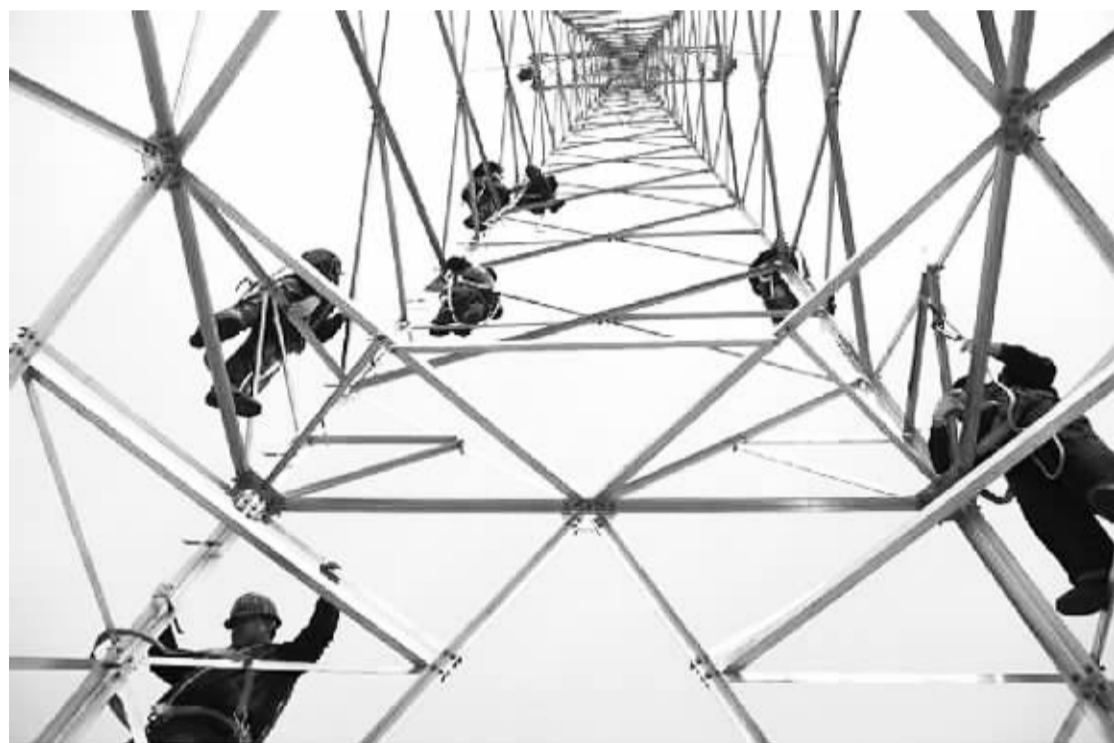
5月12日,郑州供电公司员工正在组建哈密南-郑州±800千伏特高压直流输电铁塔。哈密南-郑州±800千伏特高压直流输电工程是“疆电外送”的首个特高压项目,郑州供电公司作为其中部分项目的承建方选派精兵强将参与建设。目前,该项目正在紧张施工中,预计将于年内全线贯通。(胥培红 代锦霞)
